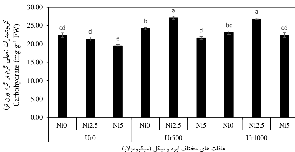
غلظت های مختلف اوره و نیکل (میکرومولار) Different concentrations of urea and nickel ( \mu\text{mol L}^{-1} )
